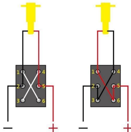
圖 2. 電流正反轉接線圖
