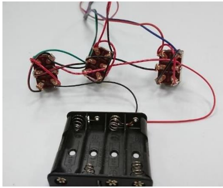
圖 4. 三顆馬達接法
