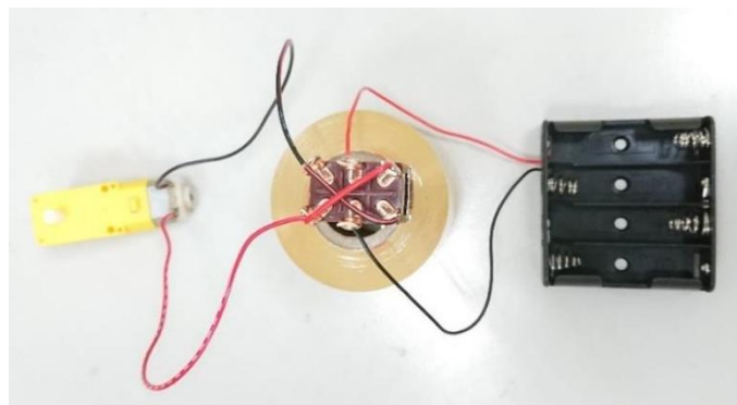
圖 3. 單顆馬達接法
